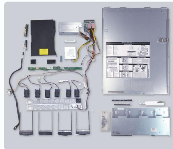
▲ 变更为液浸用服务器时不需要的部件（例）
