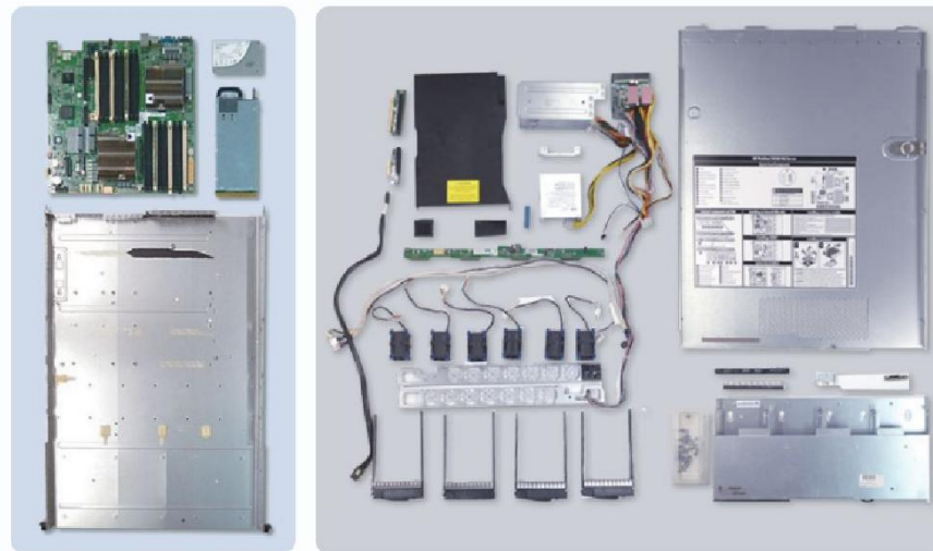
▲ 液浸用服务器部件的构成 (例) ▲ 变更为液浸用服务器时不需要的部件 (例)
